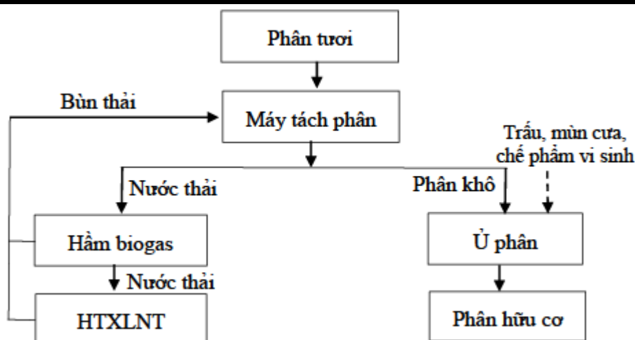
Hình 3. 11. Sơ đồ công nghệ xử lý phân tươi
