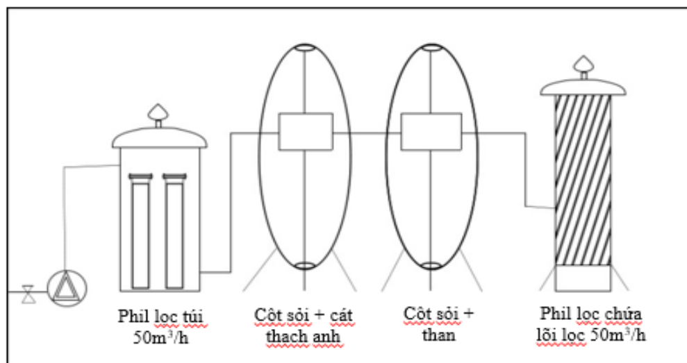
Hình 1. 10. Hệ thống xử lý nước cấp
