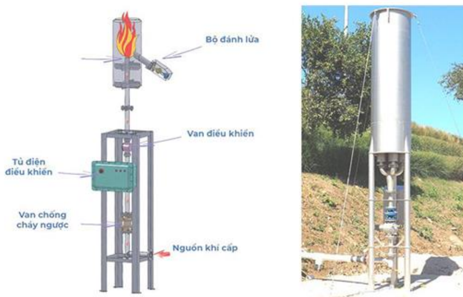
Hình 3. 12. Béc đốt khí Biogas (tham khảo)
