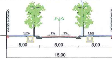
MẶT CẮT 1-1
