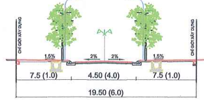
MẶT CẮT 2-2 (3-3)
