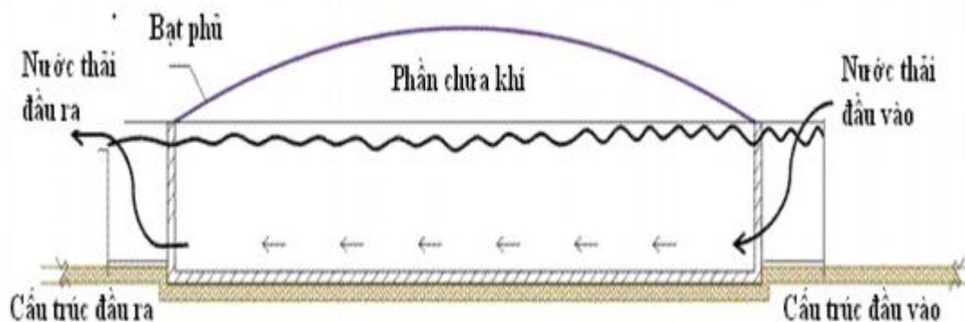
Hình 3. 7. Sơ đồ nguyên lý hoạt động của bể biogas
