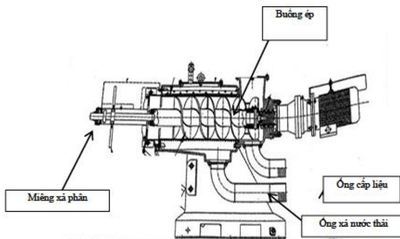
Hình 3. 10. Cấu tạo của máy ép phân
