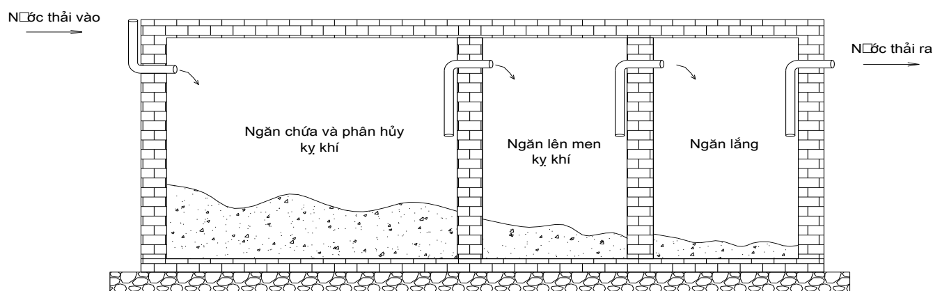
Hình 1. 6. Sơ đồ cấu tạo bể tự hoại
