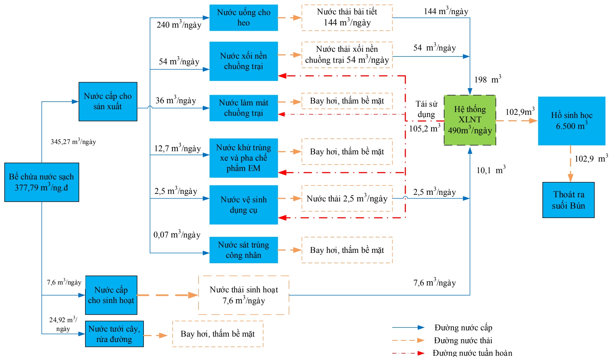
Hình 1. 9. Sơ đồ cân bằng nước của dự án mùa mưa
