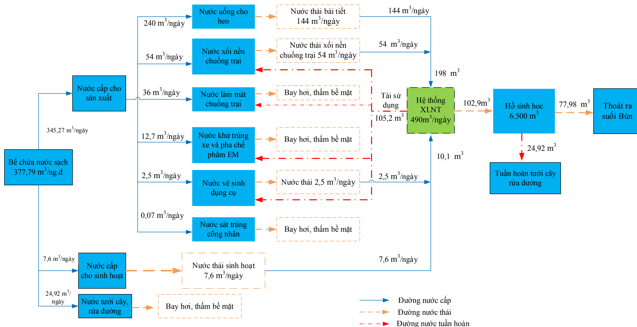
Hình 1. 8. Sơ đồ cân bằng nước của dự án mùa khô
