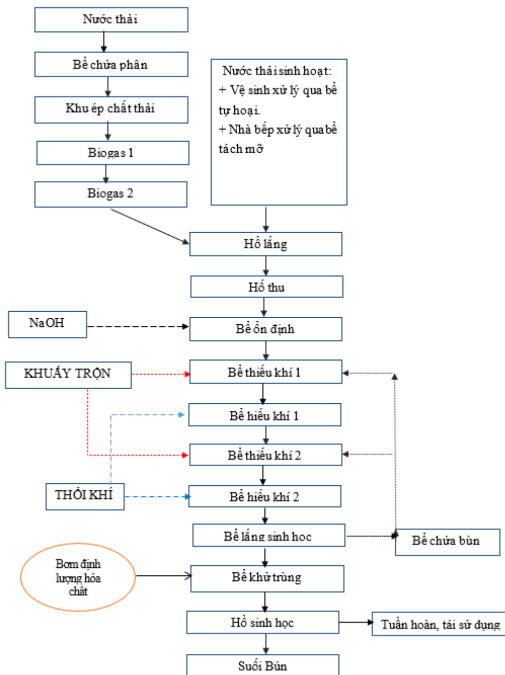
Hình 3. 6. Sơ đồ công nghệ hệ thống xử lý nước thải
