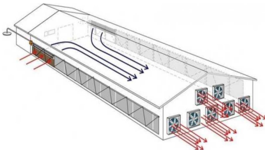
Hình 3. 8. Phương án lắp quạt thông gió cho dãy chuồng lợn
