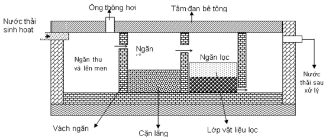
Hình 3. 5. Cấu tạo bể tự hoại
