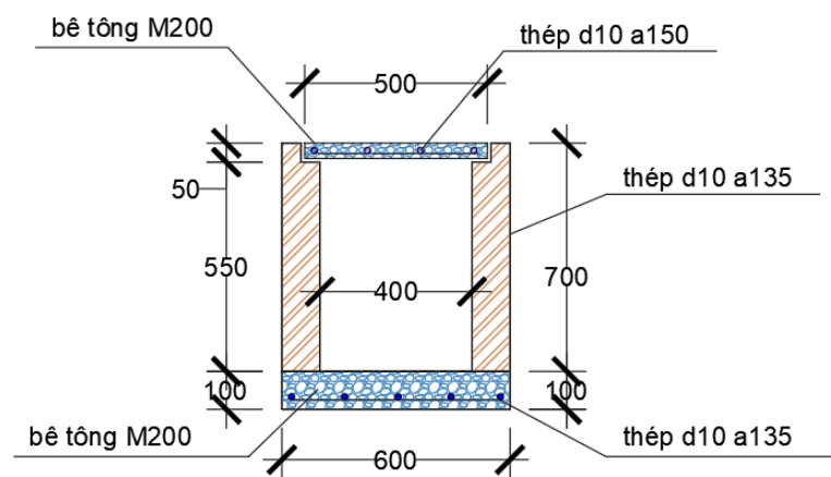
Hình 1. 5. Mặt cắt mương thoát nước
