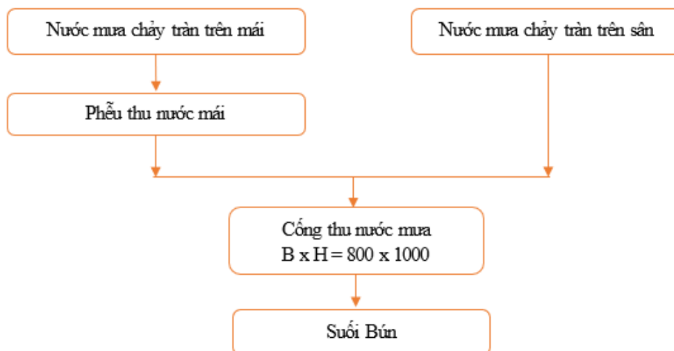
Hình 3. 4. Sơ đồ mạng lưới thu gom nước mưa
