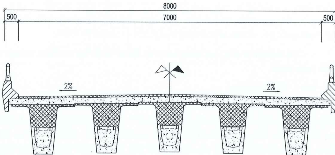
Hình 1-5: Mặt cắt ngang cầu trên tuyến
