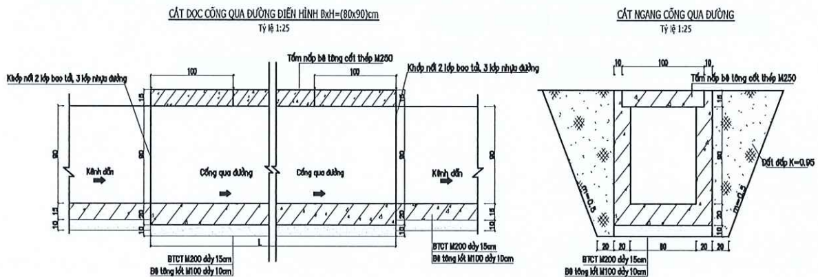
Hình 1-8: Thiết kế điển hình cống qua đường công trình I-1
