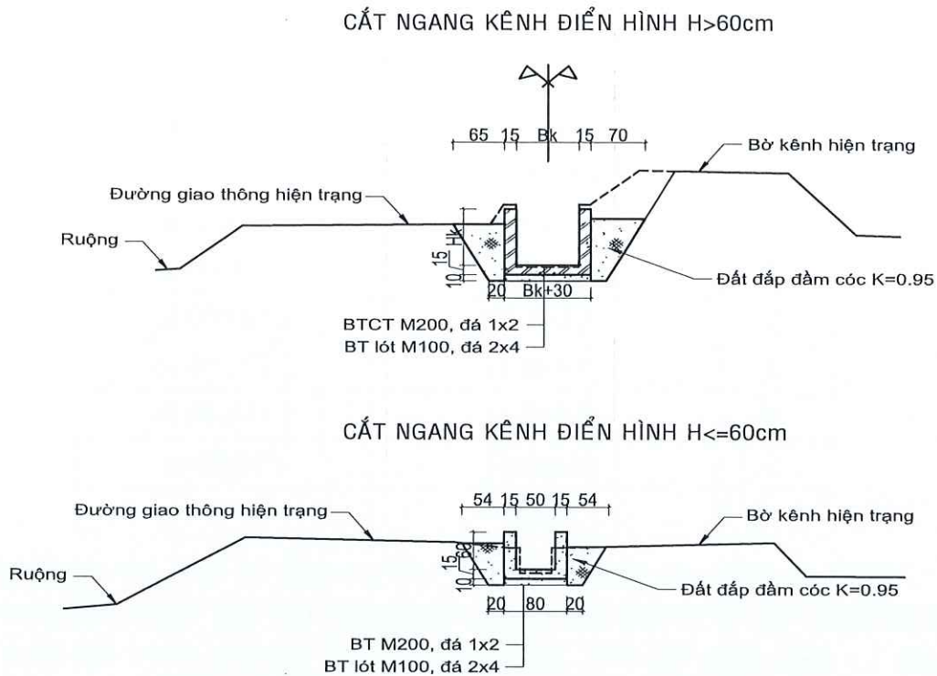
Hình 1-7: Mặt cắt ngang đại diện tuyến kênh công trình I-1
