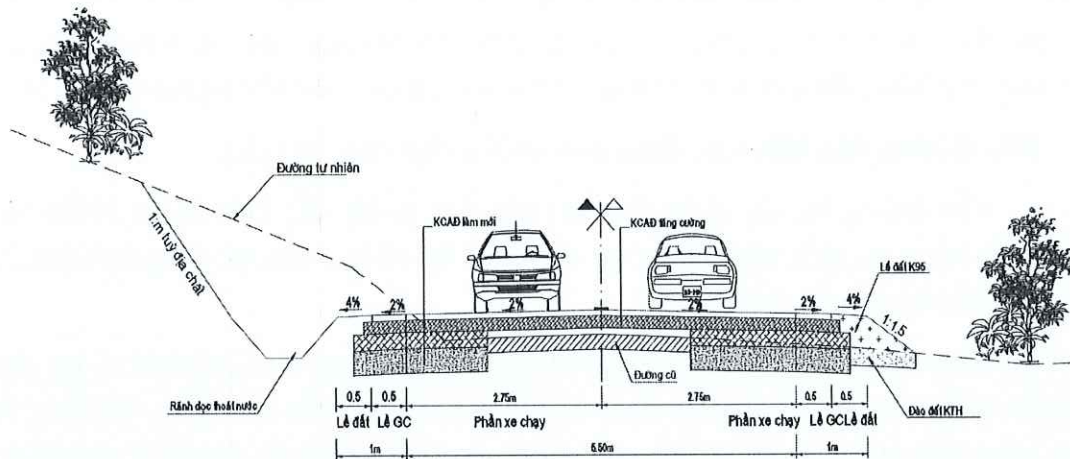
Hình 1-4: Mặt cắt ngang điển hình của DT.176B
