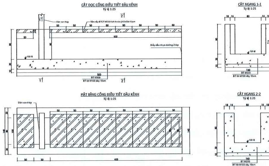
Hình 1-12: Thiết kế điển hình công điều tiết công trình I-4
