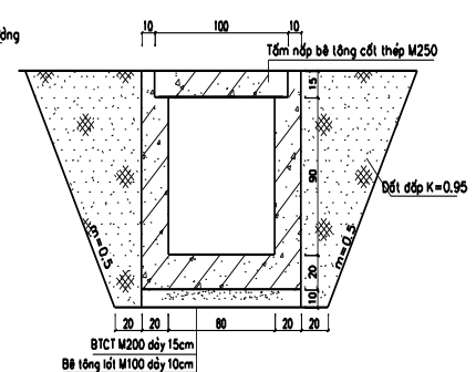
Hình 1–8: Thiết kế điển hình cống qua đường công trình I-1
