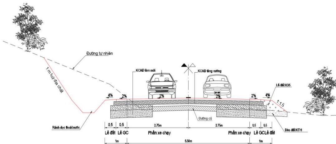
Hình 1-3: Mặt cắt ngang điển hình của ĐT.176B
