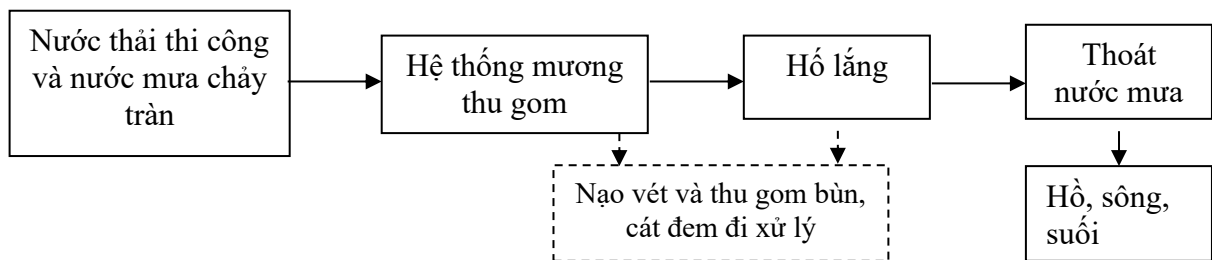
Hình 3-6: Sơ đồ xử lý nước vệ sinh từ các máy móc xây dựng
