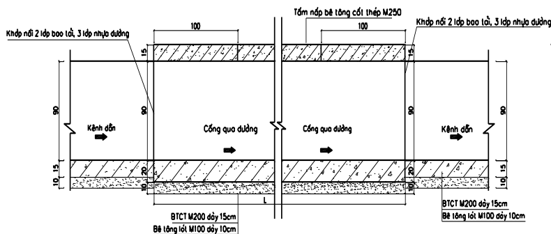
Hình 1–8: Thiết kế điển hình cống qua đường công trình I-1
