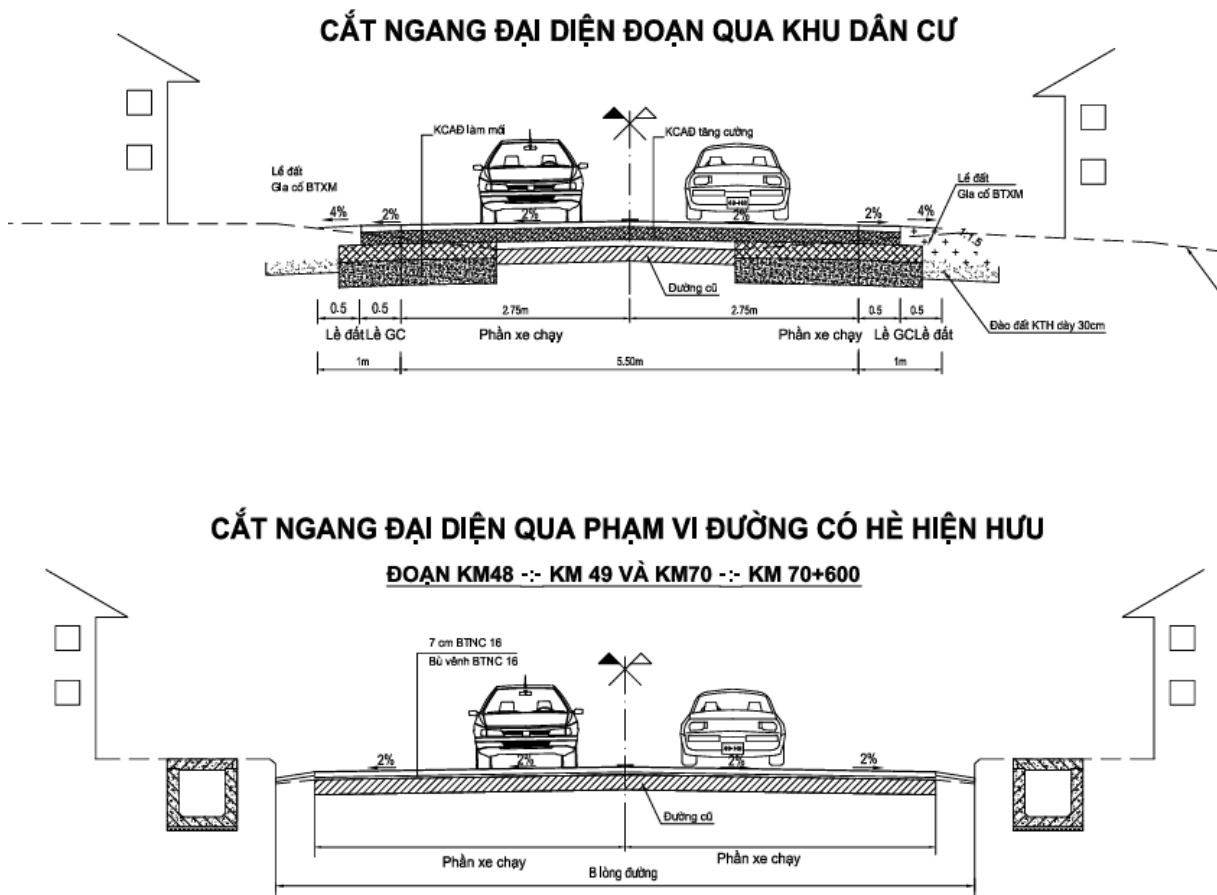
Hình 1–4: Mặt cắt ngang điển hình đường ĐT.176B đoạn có vỉa hè hiện trạng
